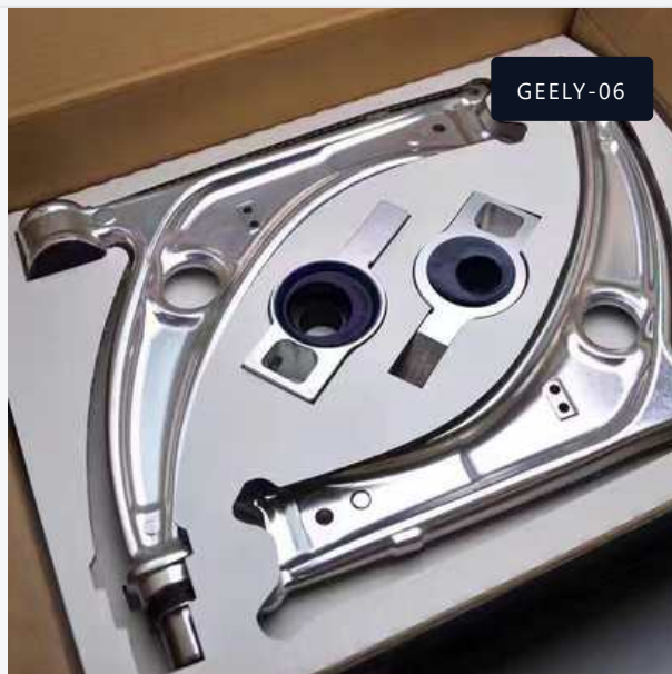
前下摆臂
